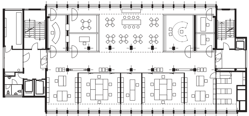
Grundriss 3. OG mit Büros, Besprechungszone «Marktplatz» und Radiostudios
